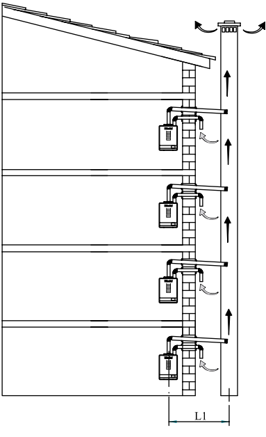
рис2 пример №2 установки общей дымоходной трубы
